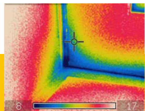
Slecht geïsoleerde houten voordeur
